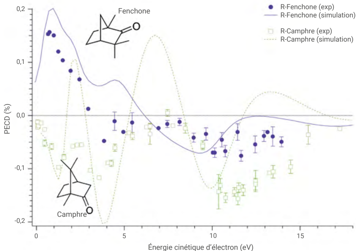
1. Sensibilité à l'isomérisation. Les PECD expérimentaux et théoriques du R-camphre (en vert) et de la R-fenchone (en bleu) diffèrent complètement, notamment pour les électrons lents, les plus sensibles au potentiel moléculaire (adapté de [11]). Dans les schémas des molécules de camphre (en bas) et de fenchone (en haut), les intersections entre les lignes représentent les atomes de carbone ; les atomes d'hydrogène ne sont pas représentés.
