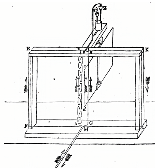
8. L'un des quatre dispositifs conçus par Ampère pour étudier l'équilibre entre conducteurs.
