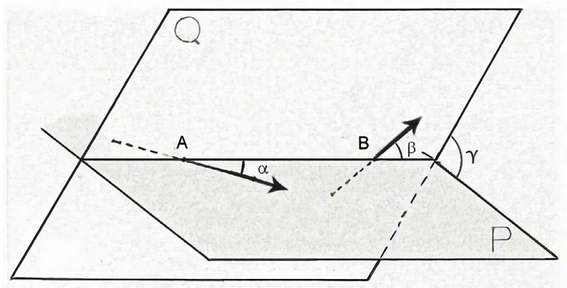
7. Configuration d'Ampère pour l'étude générale de l'interaction entre deux éléments infinitésimaux de courant, l'un centré en A, l'autre en B. ( www.ampere.cnrs.fr/ )
