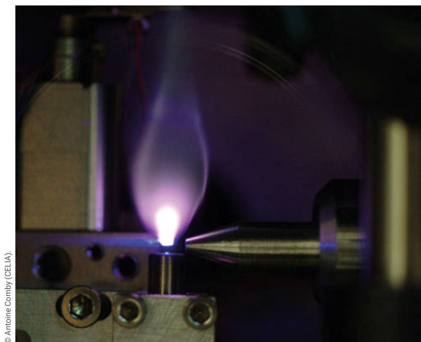
Photographie de la plume plasma créée lors de l'interaction entre le laser et le jet de gaz (voir la figure 2, p. 14). Ici, le gaz arrive par le tube vertical sous la flamme. Le laser vient de la gauche et entre dans un petit trou du tube à droite (pompage différentiel). Le filtre infrarouge et le réseau ne sont pas visibles sur la photo.
