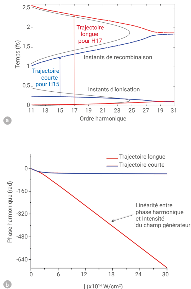
E1. (a) Tracé des temps d'ionisation (courbes pleines, t = 0 correspond au maximum du champ électrique oscillant à une période de 2,66 fs) et des temps de recombinaison (courbes en tirets) en fonction de l'ordre harmonique. Les temps d'excursion (différences entre les temps de recombinaison et d'ionisation) pour les harmoniques 17 (H17, exemple de trajectoire longue) et 15 (H15, exemple de trajectoire courte) sont indiqués. Ces temps ont été obtenus par une approche quantique, et la courbe noire en trait plein est l'équivalent obtenu par une approche classique. (b) Tracé de la phase du dipôle harmonique de H15, à titre d'exemple, obtenue par simulation en fonction de l'intensité du champ laser générateur. La relation de linéarité entre phase et intensité est clairement montrée pour les trajectoires longues, mais aussi pour les trajectoires courtes avec un paramètre de linéarité beaucoup plus petit que pour les trajectoires longues.
