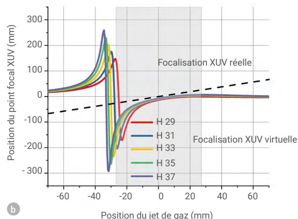
4. Simulations numériques. a) Résultats théoriques modélisant les conditions expérimentales de la figure 3c pour les trajectoires courtes. Pour les simulations, seules les trajectoires courtes (voir l'encadré, p. 13) sont considérées. b) Simulations de la position du point focal des harmoniques, décrites par des faisceaux gaussiens, en fonction de la position du jet de gaz. Les conditions de génération sont identiques à celles de la figure 4a. La ligne en tirets sépare la zone où les harmoniques sont focalisées après la génération (focalisation réelle) de la zone où elles semblent provenir d'un point focal situé en amont de la génération (focalisation virtuelle).
