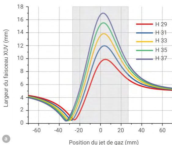
4. Simulations numériques. a) Résultats théoriques modélisant les conditions expérimentales de la figure 3c pour les trajectoires courtes. Pour les simulations, seules les trajectoires courtes (voir l'encadré, p. 13) sont considérées. b) Simulations de la position du point focal des harmoniques, décrites par des faisceaux gaussiens, en fonction de la position du jet de gaz. Les conditions de génération sont identiques à celles de la figure 4a. La ligne en tirets sépare la zone où les harmoniques sont focalisées après la génération (focalisation réelle) de la zone où elles semblent provenir d'un point focal situé en amont de la génération (focalisation virtuelle).
