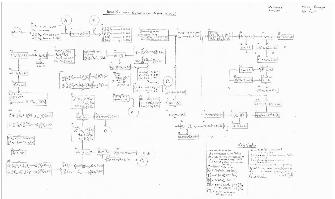
2. L'algorithme utilisé par Mary Tsingou pour coder la première expérience numérique et retrouvé dans sa cave. Notez la date du rapport de Los Alamos, 5-20-55, dans le coin en haut à droite, ainsi que le titre "New Nonlinear Vibrations – Short Method".
