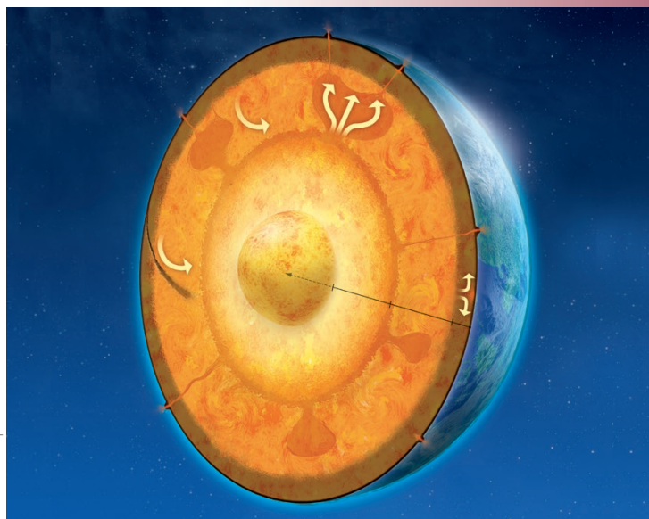
Anatomie de la Terre : la graine au centre, puis le noyau liquide, le manteau inférieur et enfin le manteau supérieur. © CNRS Photothèque - DIdéAN Anroine
