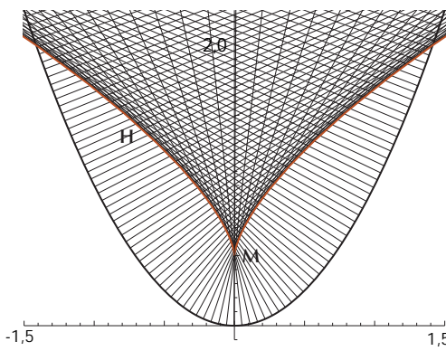
3. La construction de Bouguer :
